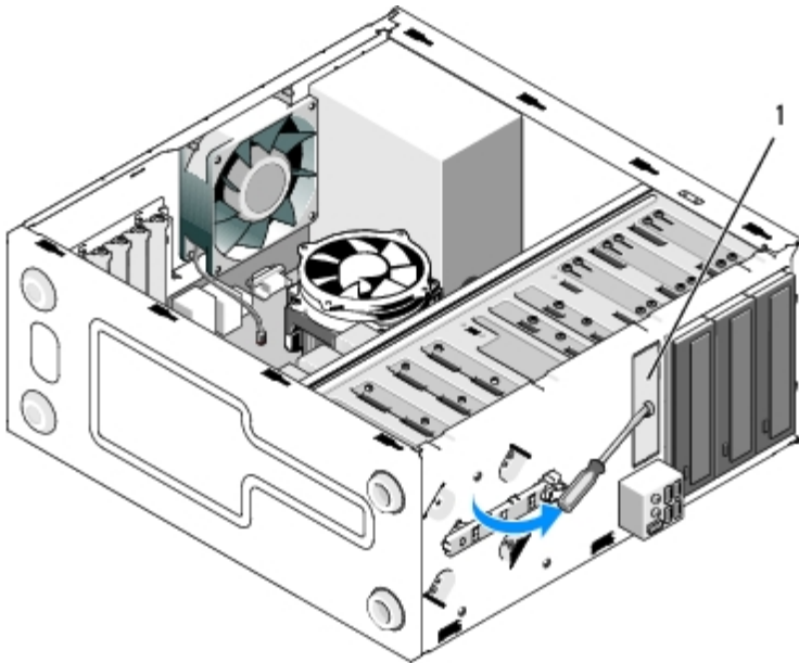
1 metalen plaatje van 3,5-inch compartiment
